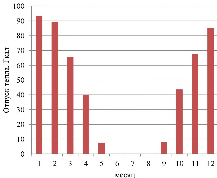
Рисунок 1.2 – Оптимальный температурный график отпуски тепловой энергии для Котельной с. Скопино
