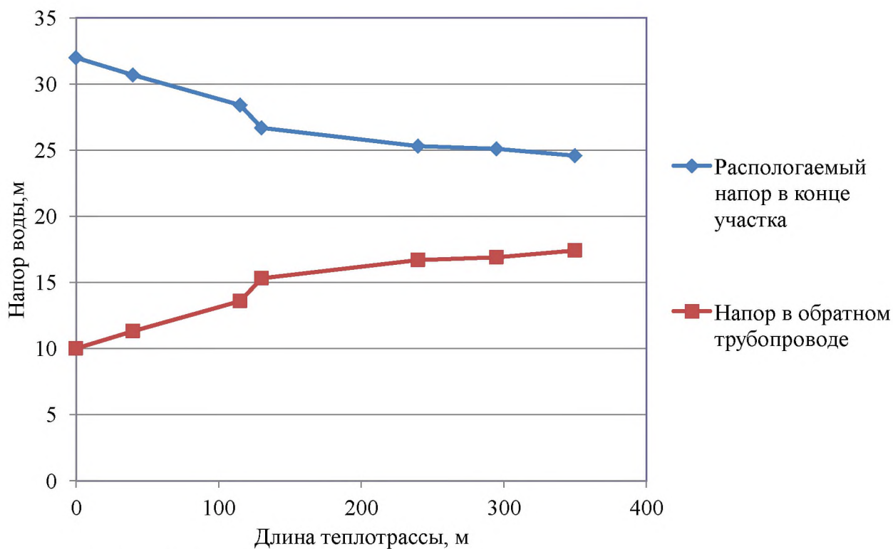
Рисунок 2.5 – Пьезометрический график тепловой сети котельной с. Скопино от котельной до детского сада
