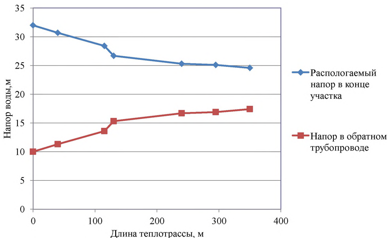
Рисунок 2.4 – Пьезометрический график тепловой сети котельной с. Скопино от котельной до детского сада
